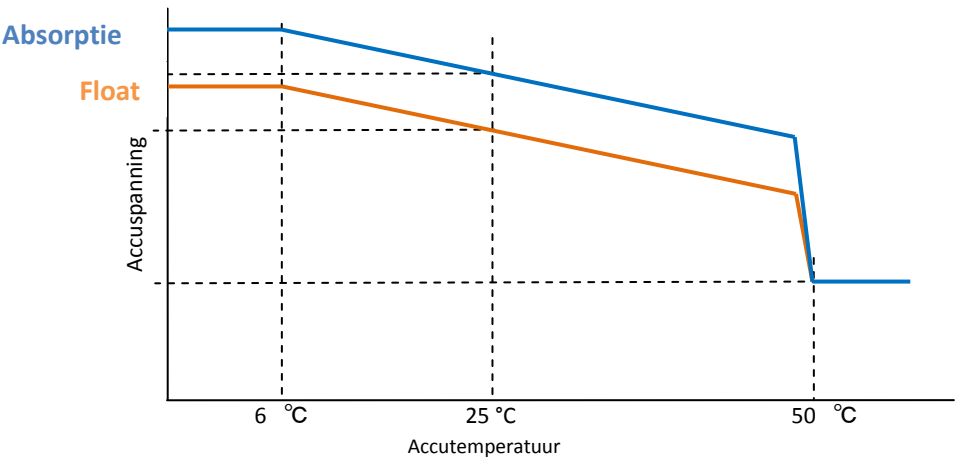
Afbeelding 1: temperatuurcompensatiecurve
